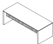
FS2000 200 - 90 - 74 FS2200 220 - 90 - 74
